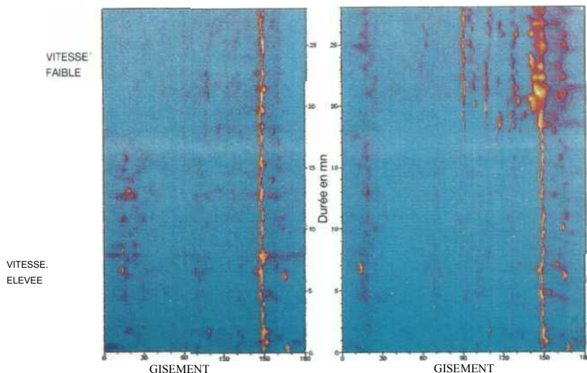
Influence du modèle de bruit sur les résultats du goniomètre.
