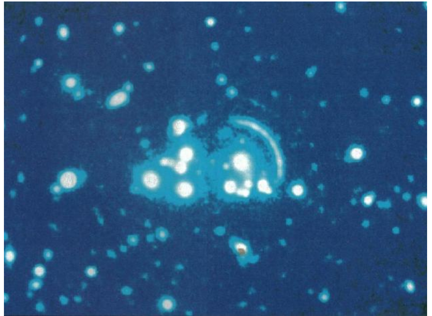
Fig. 1 - Image CCD ultraprofonde dans le centre de l'amas C12244. Pour la population de galaxies bleues, la composante de matière invisible et de nature inconnue qui domine le potentiel de l'amas, forme des arcs gravitationnels sur le plan du ciel (cliché CFHT, octobre 1990).
