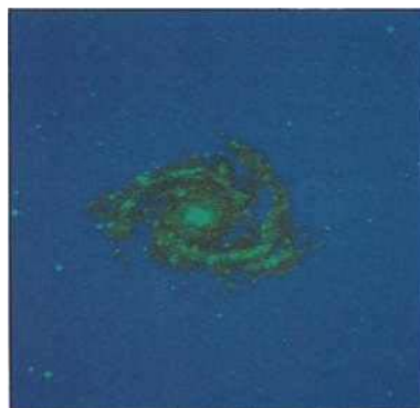
Galaxie spirale du ciel austral: après de la MAMA sont entreposées les copies sur verre des relevés du ciel sud, réalisés avec un filtre rouge à l'Observatoire européen austral, et avec un filtre bleu à l'observatoire britannique de Siding Springs (Australie). Les régions d'hydrogène ionisé par les étoiles chaudes récemment formées sont bien visibles le long des bras spiraux de cette galaxie photographiée à Siding Springs et numérisée avec la MAMA.
