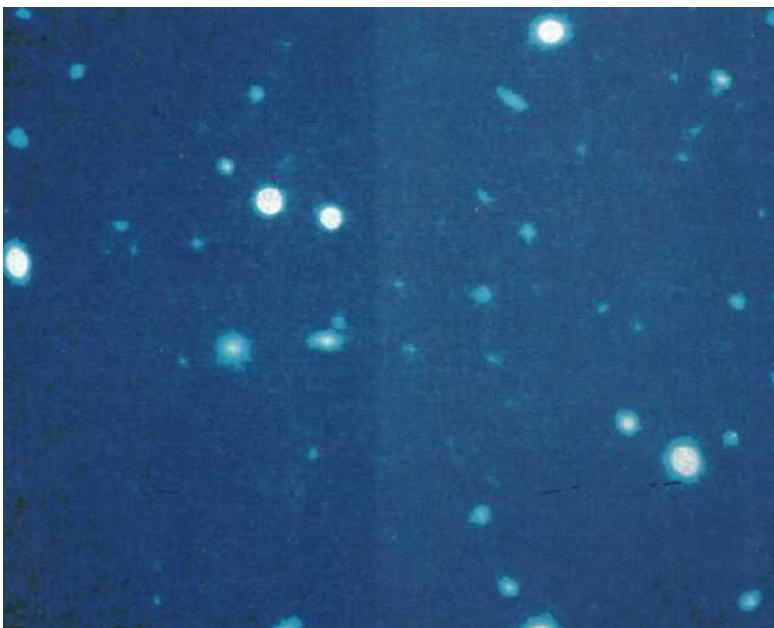
Fig. 2- Image CCD ultraprofonde d'un champ présumé vide d'objets sur le Palomar sky survey. On y distingue la population de galaxies bleues distantes de plus de dix milliards d'années-lumière dont la brillance est inférieure au centième du fond du ciel (cliché CFHT, octobre 1990).
