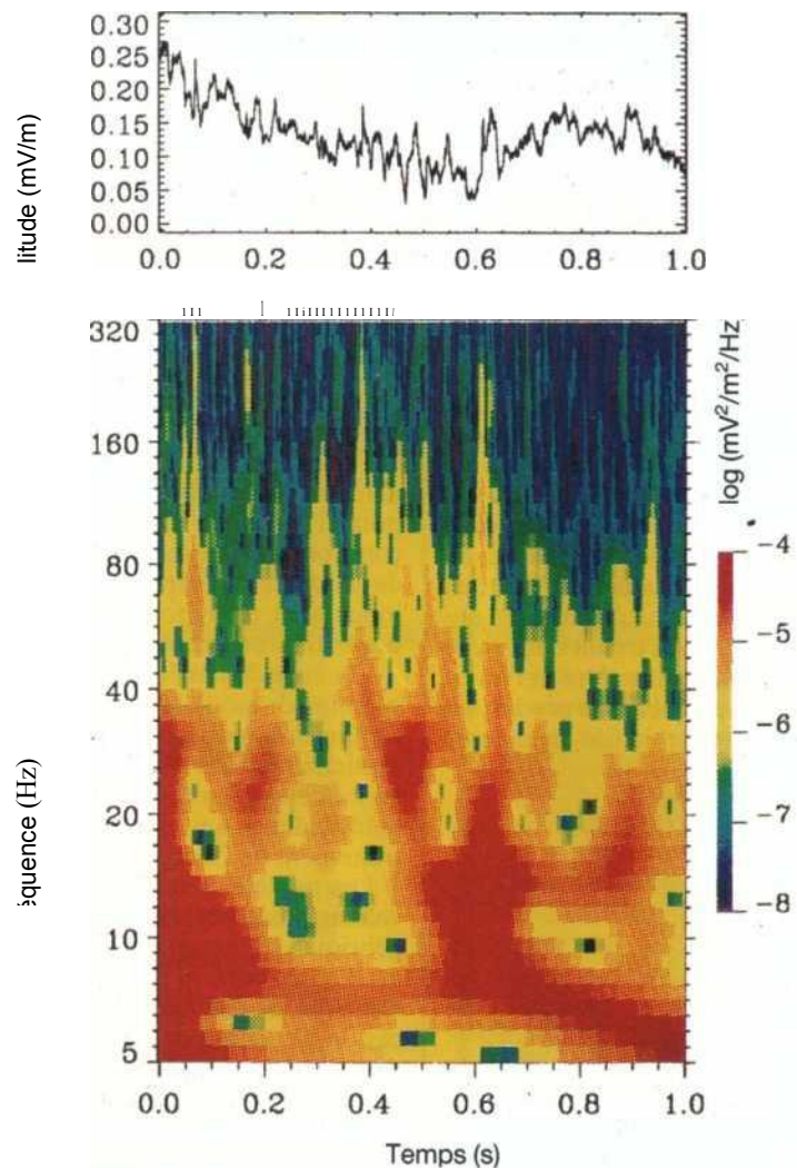
Forme d'onde (haut de la figure) et module de la transformée en ondelettes (bas de la figure) d'une composante du champ électrique mesuré dans l'ionosphère terrestre. La finesse des structures verticales est à la limite de la résolution de l'analyse, ce qui indique la faible cohérence spatio-temporelle de la turbulence.
