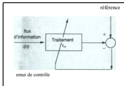
Fig. 1 - Traitement adaptatif. n = \text{temps} .
