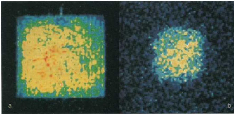
I Fig. 1 - Séchage de la pierre de Caen ; images RMN de l'eau dans une pierre calcaire de porosité 25 % en cours de séchage. La pierre est un cube de 10 cm de côté. Elle est saturée en eau puis progressivement séchée et examinée par imagerie RMN. Entre les deux images, les conditions d'acquisition sont identiques sauf la saturation en eau S = 33\% (figure a) et S = 4\% (figure b). Les images représentent une tranche d'épaisseur 8mm, et elles montrent que la répartition de l'eau dans le cube reste quasi uniforme pour S = 33\% tandis que pour S = 4\% , l'eau résiduelle est concentrée au centre de la pierre. Ceci s'explique par la valeur relative de S par rapport à la saturation irréductible qui est de l'ordre de 20%. Pour S = 33\% , la phase liquide a une bonne connectivité dans le matériau poreux qui maintient une perméabilité élevée donc une répartition rapide de l'eau malgré l'évaporation à l'extérieur de la pierre. Par contre, en dessous de la saturation irréductible, la perte de connectivité de la phase liquide empêche la réuniformisation de la distribution de l'eau. (La résolution dans le plan de l'image est 2 \times 2 \text{ mm}^2 Le temps d'acquisition est de 15 minutes environ). (D'après G. Guillot, A. Trokiner, L. Darrasse et H. Saint-Jalmes)
