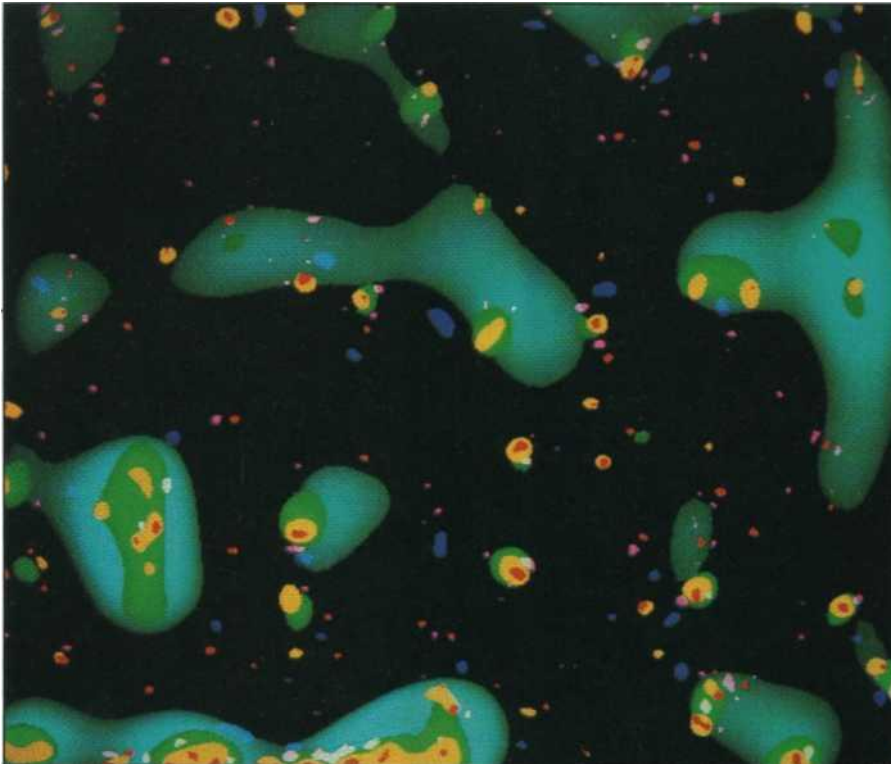
Hierarchie des structures observées à partir d'un comptage de galaxies dans la constellation de la Chevelure de Bérénice . On ne visualise en fausses couleurs que les coefficients en ondelettes dont le degré de signification statistique est supérieur à 99,9% pour quatre échelles croissant du rouge au jaune, vert, et cyan.
