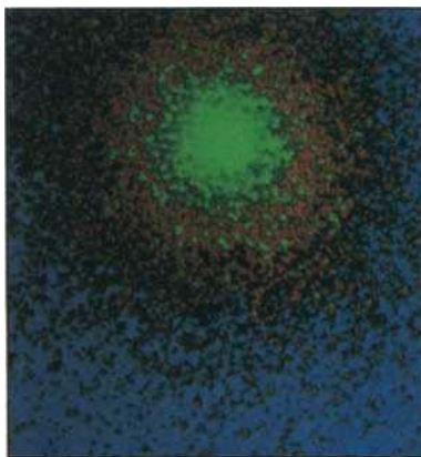
Amas globulaire Messier 5 : la calibration photométrique des clichés photographiques repose souvent sur l'utilisation de séquences d'étoiles situées dans le voisinage d'amas. (Cliché Schmidt O. C. A, numérisation MAMA).
